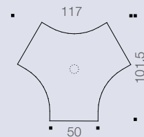
Plan de liaison triangle pour 3 tables rectangulaires, muni d'1 passe-câble pré-débouchant
